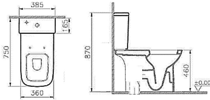
Şekil 3. A firmasına ait A1 Klozet
