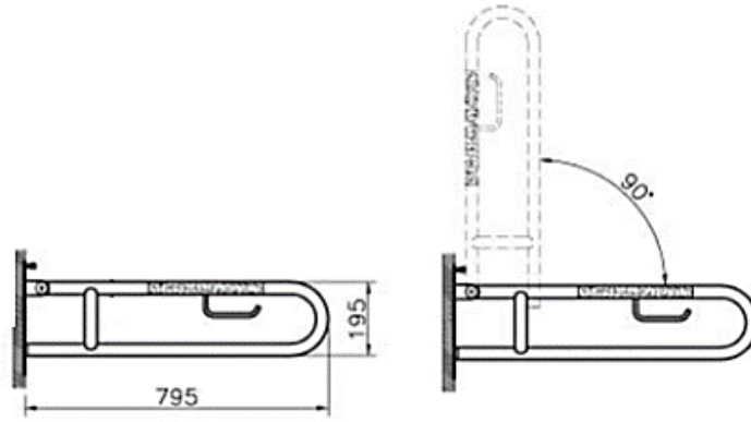
Şekil 29. A firmasına ait A2 Katlanabilir Tutunma Barı
