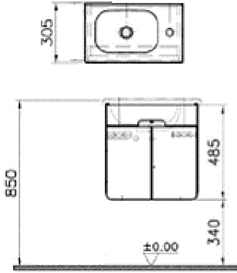
Şekil 45. A firmasına ait A8 Lavabo Dolabı
