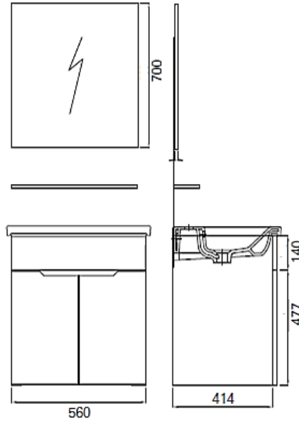
Şekil 55. D firmasına ait D7 Banyo Mobilyası
