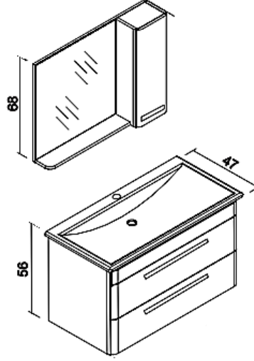
Şekil 63. E firmasına ait E2 Banyo Mobilyası
