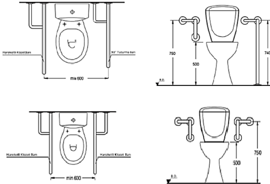
Şekil 31. B firmasına ait B1 Hareketli Klozet Barı
