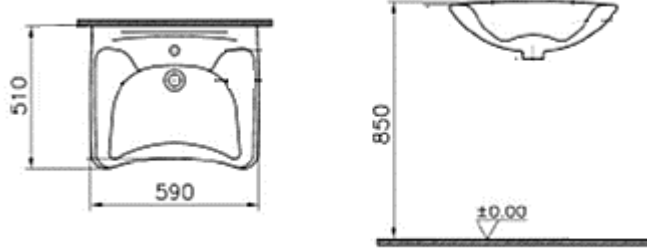
Şekil 18. A firmasına ait A2 Lavabo
