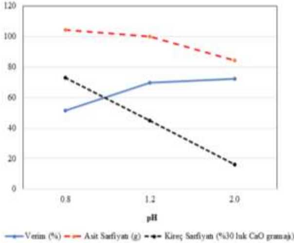
Şekil 5. Zn çözünme verimi, asit sarfiyatı ve nötralleştirme için gerekli kireç miktarına pH'ın etkisi.
