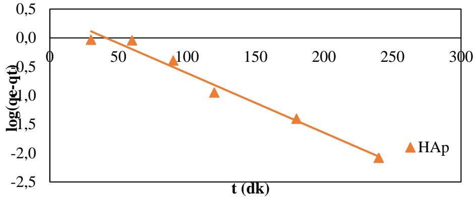
Şekil 6.10 Kristal Viyole adsorsiyonun Yalancı birinci dereceden kinetiği
