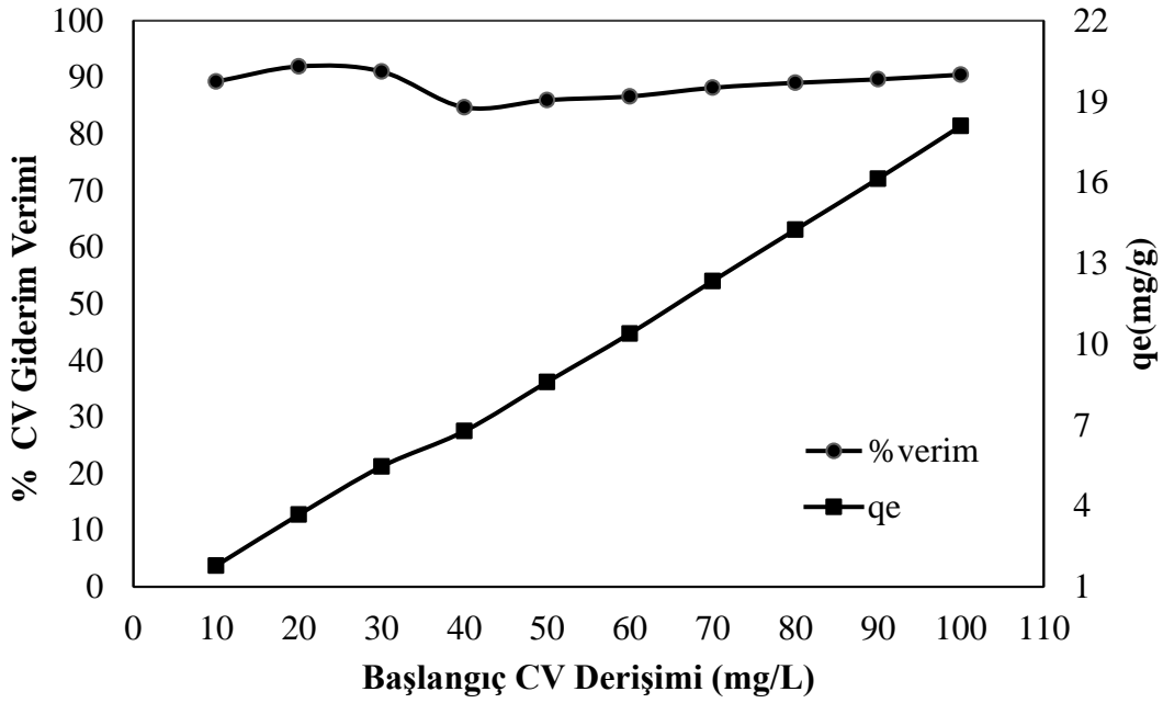
Şekil 6.2 HAp'in CV gideriminde çözelti derişimin etkisi (m:0.5 g, pH:4, T:25 °C, 300 rpm ve 120 dk).
