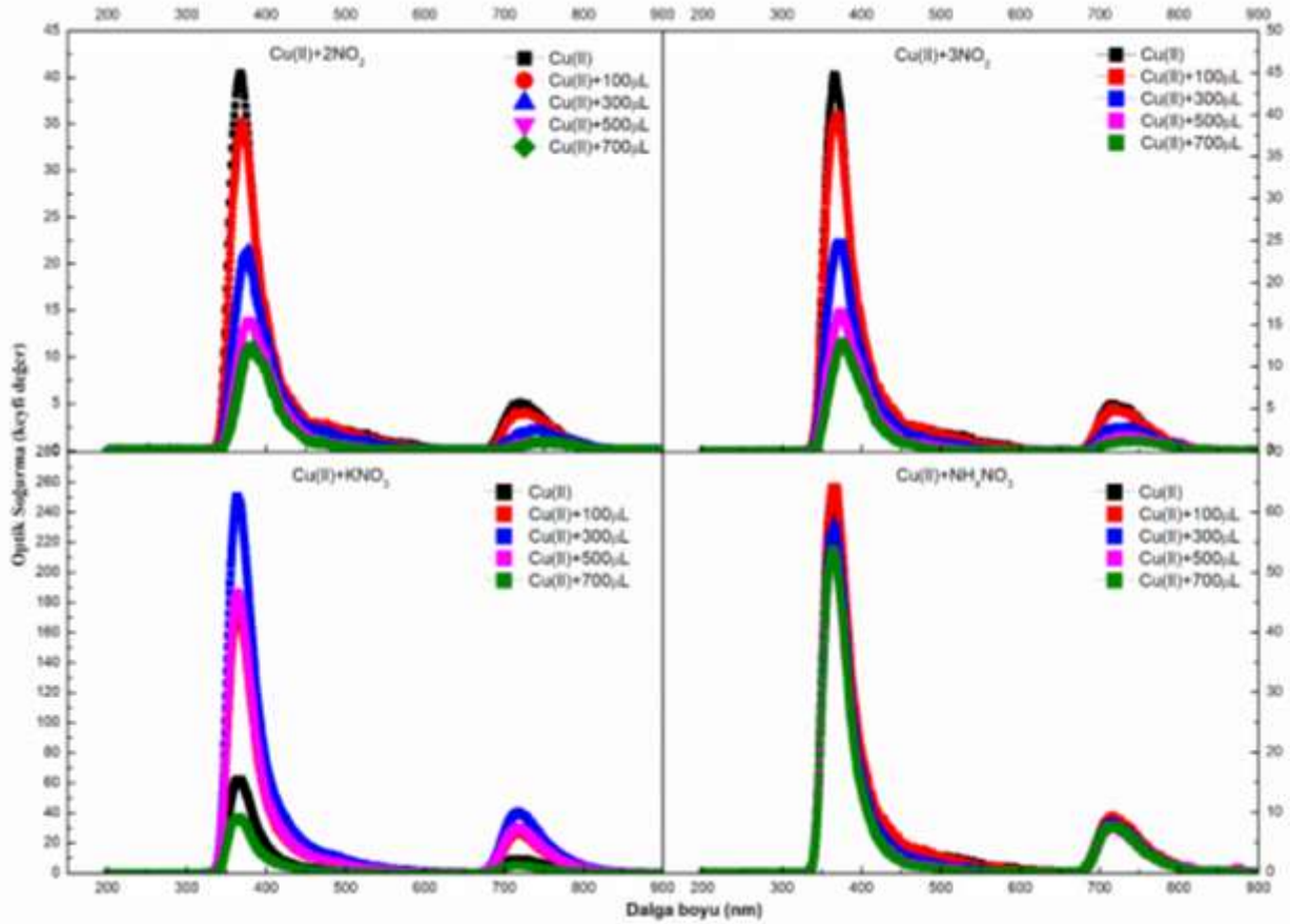
Şekil 2. Cu(II) kompleksi ve içerisinde 2NO_2 , 3NO_2 , KNO_3 ve NH_4NH_3 eklenmiş hallerinin optik soğurma spektrumları.
