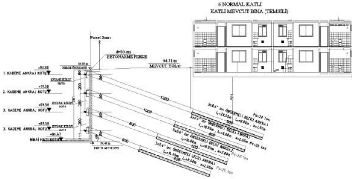
Şekil 1.1. Tipik bir Ankrajlı Betonarme Perde Duvar ( ABPD) Kesiti
