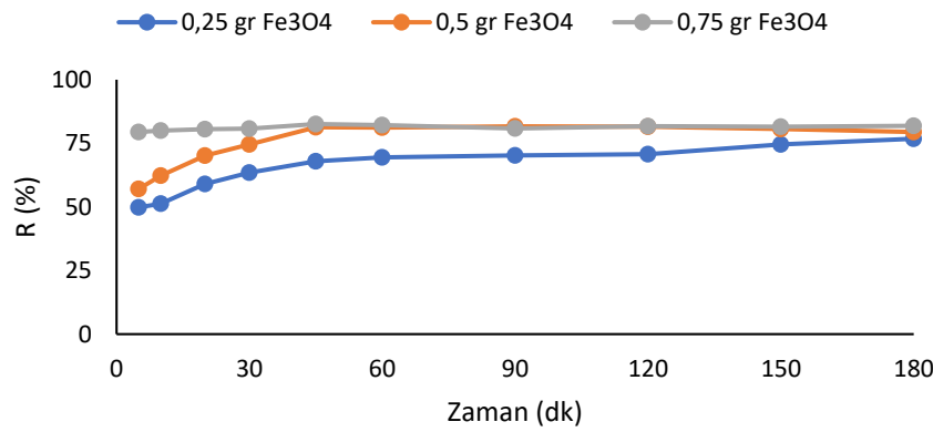
Şekil 2. Adsorbent dozajına bağlı olarak giderim verimindeki değişim ( C_o= 25 mg/L, m/V= 0,25-0,5-0,75 g/100 mL, 30^\circ\text{C} , çözelti pH değeri, 125 rpm)
