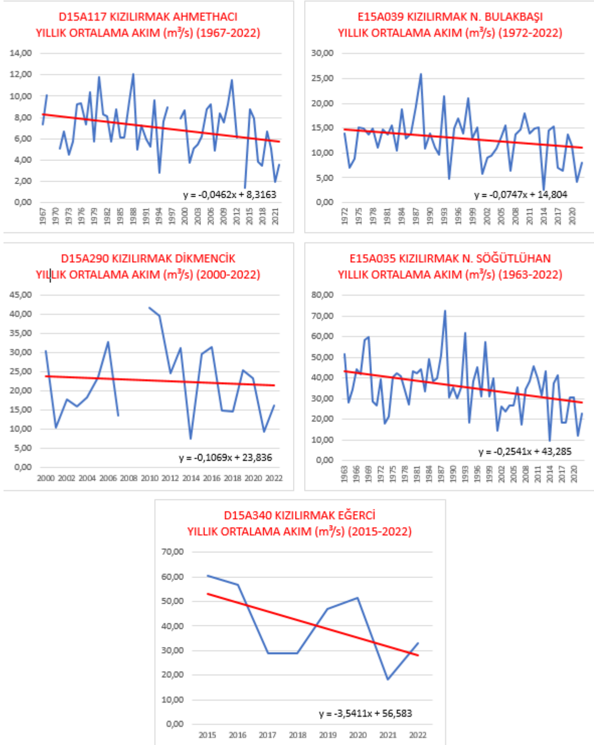
Şekil 10. Sivas Kızılırmak nehrinin Akım gözlem istasyonlarına ait ortalama akım değerleri.
