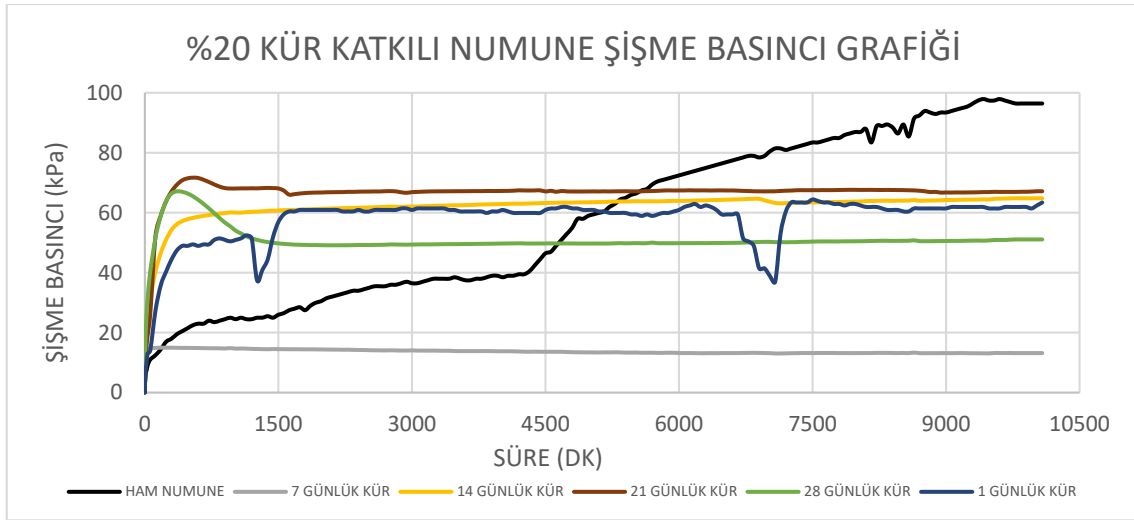
Şekil 12. %20 Kür Katkılı Numune Şişme Basıncı Grafiği
