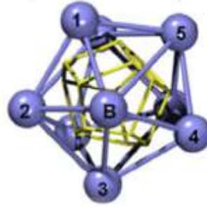
Şekil 1. VÇ'nin şematik diyagramı \langle 0, 3, 6, 0 \rangle Voronoi hücresi ve \langle 0, 3, 6, 0 \rangle VÇ ile ilişkili atomik topağı.
