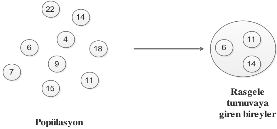
Şekil 7. Turnuva Seçilim Yöntemi
