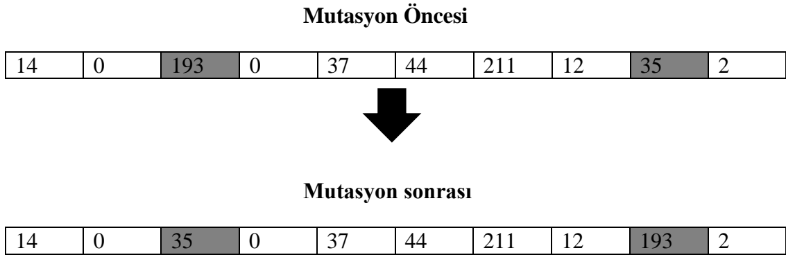
Şekil 18. Mutasyon Operatörünün Uygulanması
