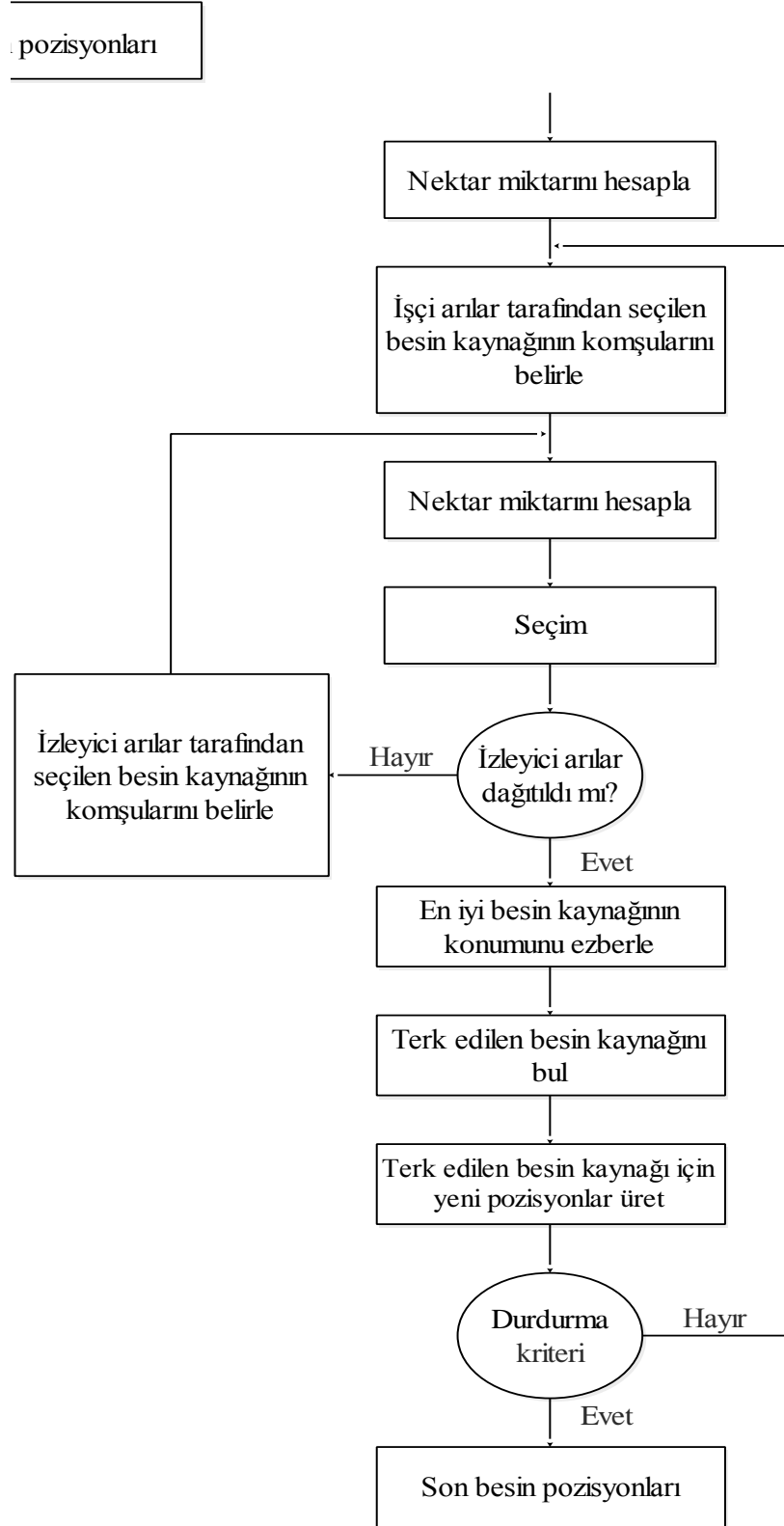
Şekil 16. ABC Algoritması Akış Diyagramı
