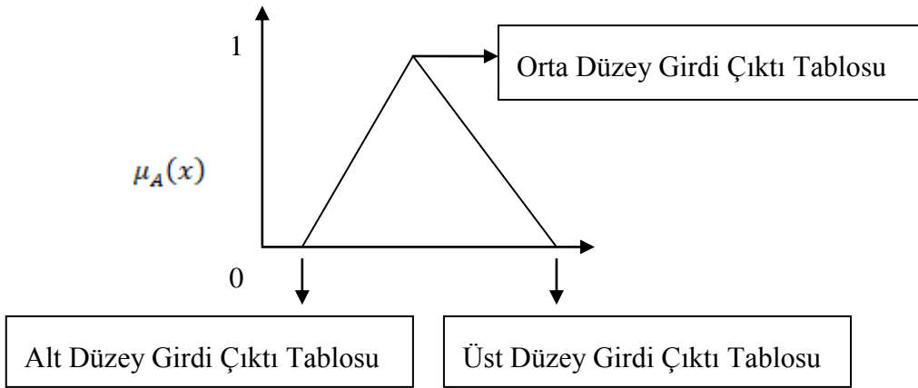
Şekil 3.8 Bulanık Girdi Çıktı Doğrusal Programlama Çözümü
