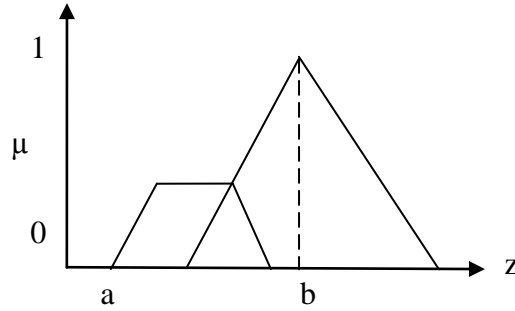
Şekil 3.5 Ağırlık Ortalaması Yöntemi
