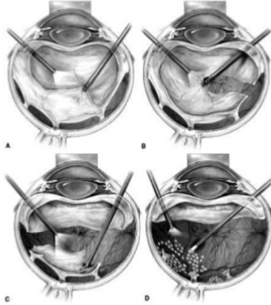
Şekil 1.13. Segmentasyon (Srivastava 2014: 41)
