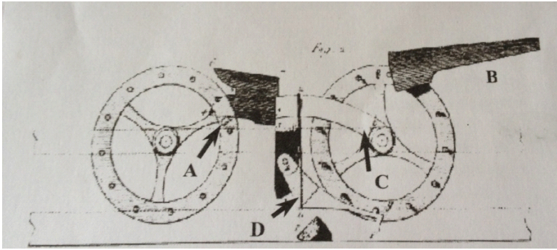
Şekil 5: İletme mekanizması
