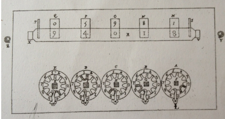
Şekil 4: Hesap makinesinin üstten görüntüsü
