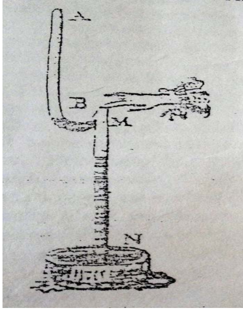
Şekil 1 : Pascal' ın tarihi vakum deneyi
