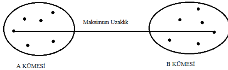
Şekil 2.6. Tam Bağlantı Yöntemi
