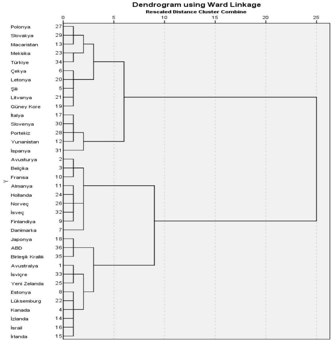
Şekil 3.5. 2019 Yılı İçin Ward Yöntemiyle Oluşturulan Dendrogram
