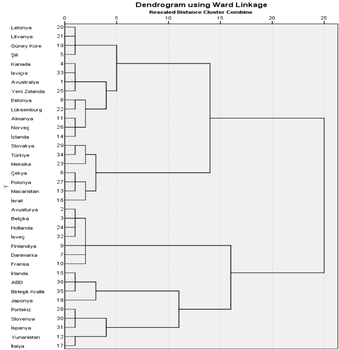
Şekil 3.3. 2017 Yılı İçin Ward Yöntemiyle Oluşturulan Dendrogram
