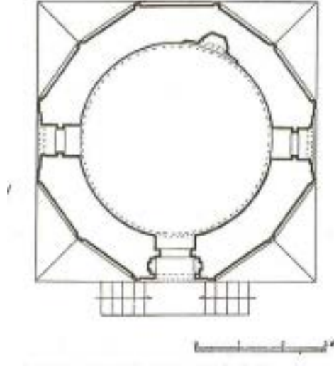
Çizim 7: Döner Kümbet Planı (Önkal 1996)
