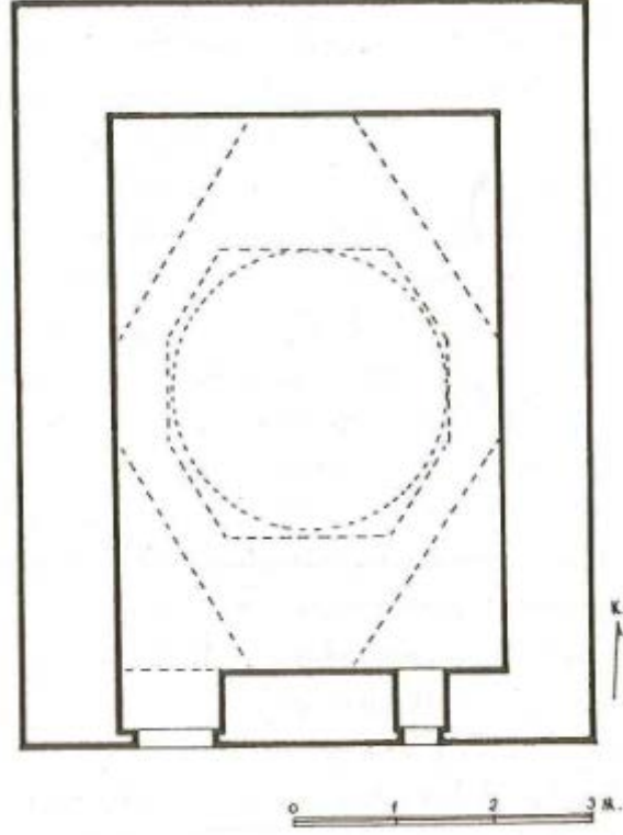
Çizim 25: Kayseri Sancaktar Türbesi Planı (Önkal 1996)
