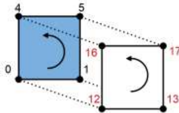
Şekil 15. Blok Oluşturmak İçin Noktaların Yazılış Sırası
