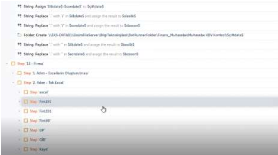
Şekil 6: GİB ve DP sistemlerine girmeyi sağlayan kod
