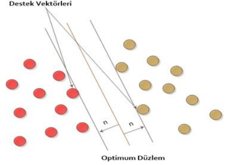
Şekil 3. Destek vektör makinesinin şeması
